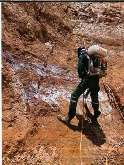
Aplicação de polímero acrílico – Coqueirinho.
