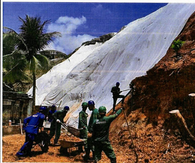
Aplicação de Geocomposto PVC – Coqueirinho.
