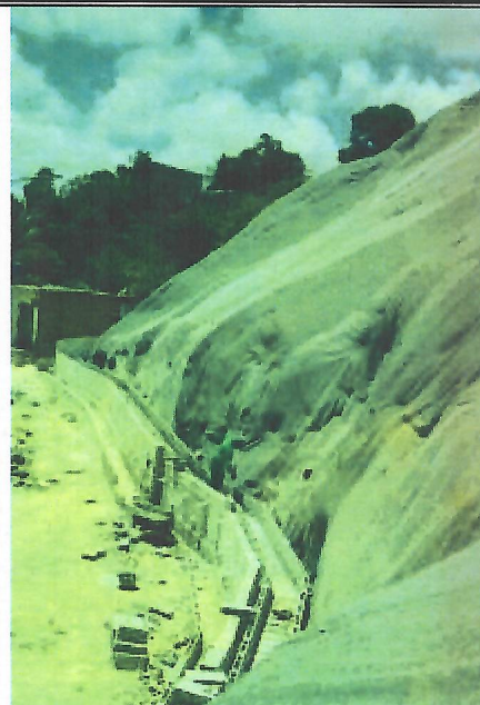
Rua 29 com 30 – Execução da canaleta 40x23 atrás e na frente do muro de flexão.
