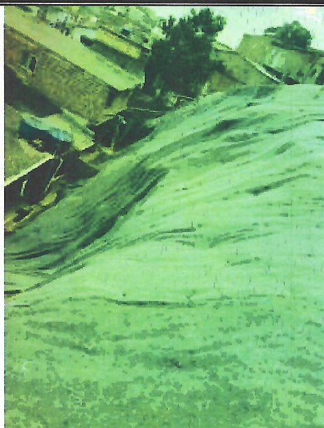
Rua Jornalista José dos Santos (talude 02) – Fornecimento e aplicação de geocomposto PVC.
