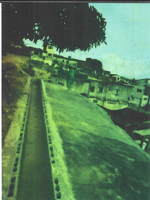
Rua 20 com 21 – Execução de canaleta 40x40.
