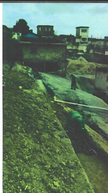
Rua 20 com 21 – Escavação manual da canaleta 40x40.
